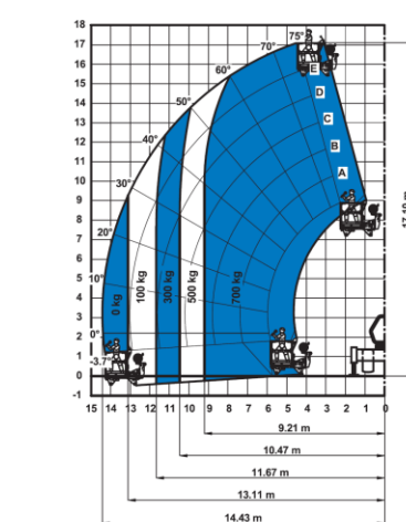
Na stabilizatorach z obrotową platformą
