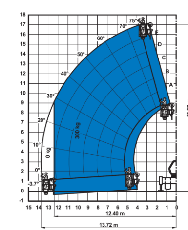
Na stabilizatorach z nieruchomą platformą roboczą
