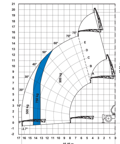
Na stabilizatorach, żuraw 900 kg (wersja mechaniczna/hydrauliczna)
