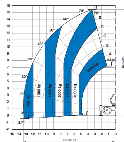
Na stabilizatorach z widłami
