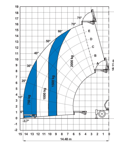
Na stabilizatorach z żurawiem 2m/1 250 kg
