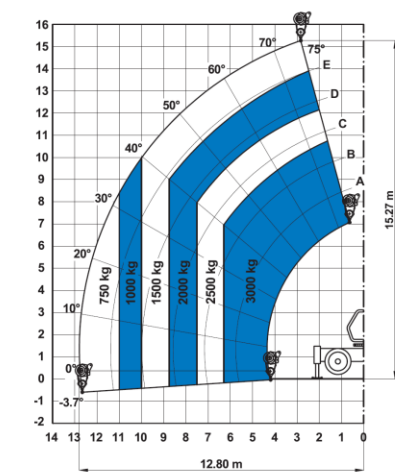
Na stabilizatorach ze wciągarką hydrauliczną
