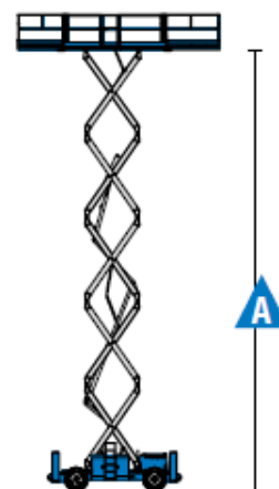
Wymiary GS-3390RT;GS-4390RT;GS-5390RT
