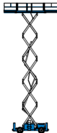
Wymiary GS-3390RT;GS-4390RT;GS-5390RT
