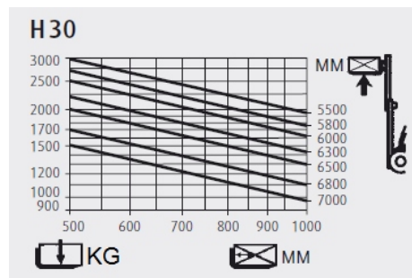
wykresy udźwignów
