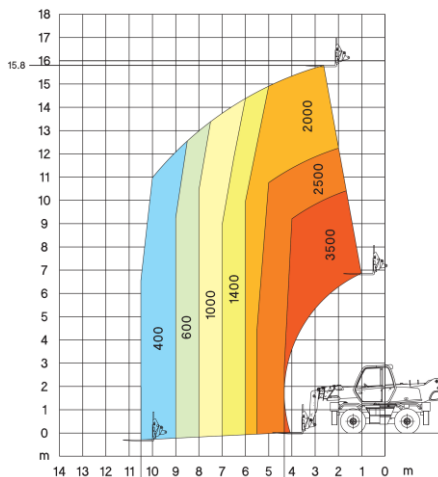
Zakres dopuszczalnych obciążeń na kołach z widłami
