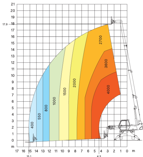
Zakres dopuszczalnych obciążeń na podporach z wciągarką 1 500 kg
