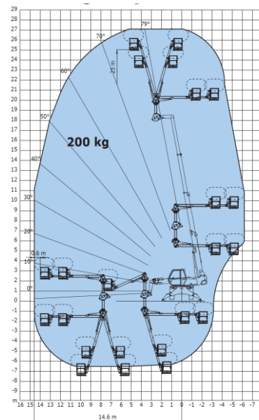
Zakres dopuszczalnych obciążeń na podporach kosz roboczy na przedłużeniu (JiB2) 200 kg - 2 osoby
